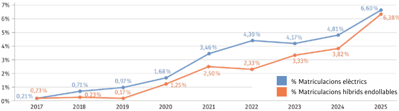
(Evolució de la proporció de noves matriculacions de vehicles que són elèctrics o híbrids endollables a l'Alt Empordà, període 2017-2025)
