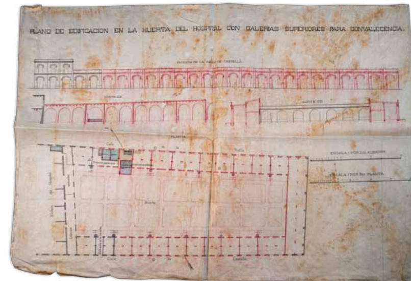
Projecte arquitectònic de Martí Sureda de l'any 1882. ACAE.
